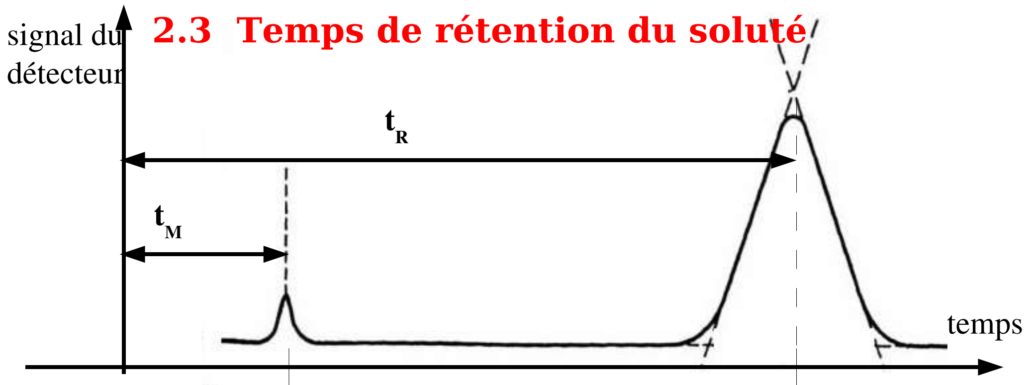
Fig. Courbe d'élution ou Chromatogramme d'un mélange à 2 constituants
