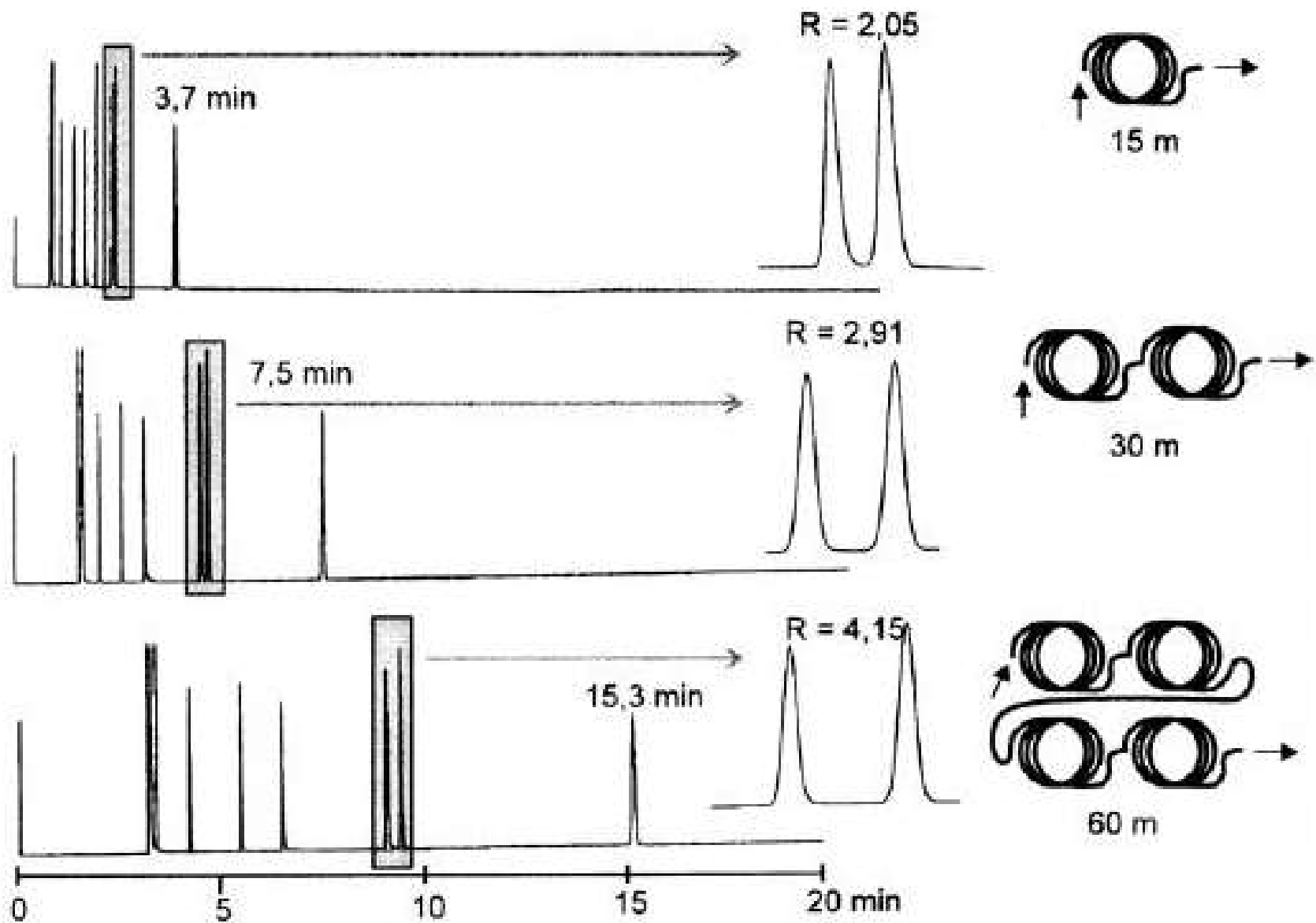
Fig. Effet de la longueur d'une colonne CPG sur la résolution
