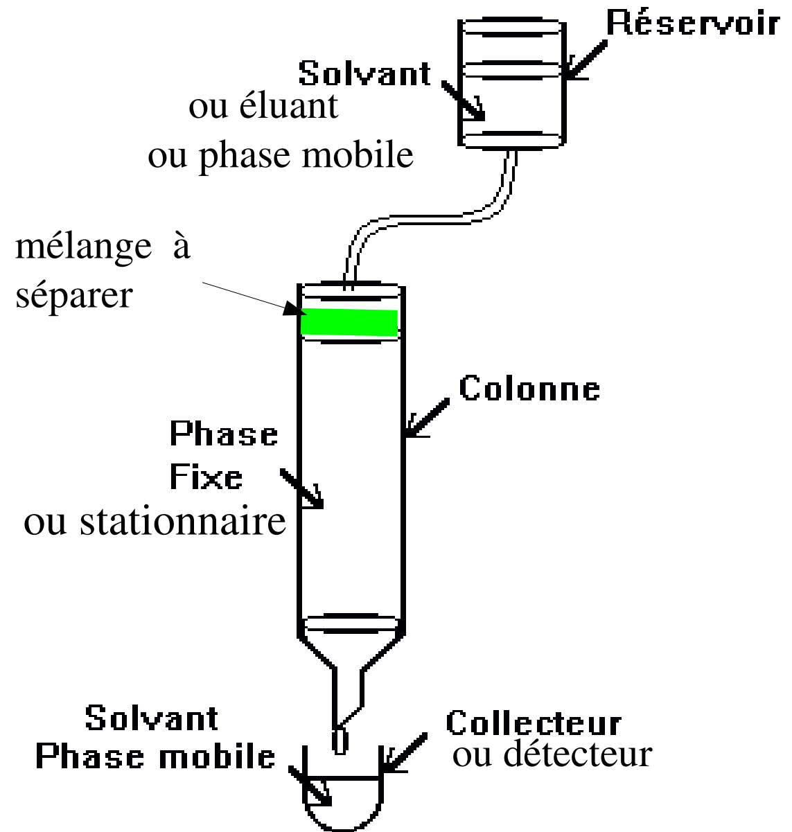
Fig. Chromatographie d'élu tion sur colonne
