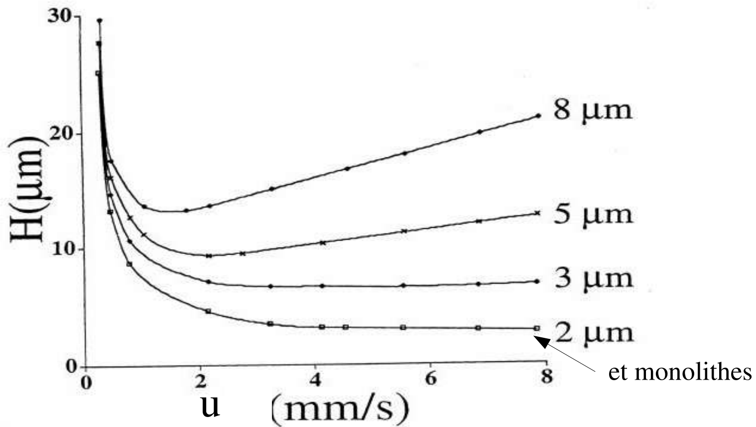
Fig. Hauteur équivalente à un plateau théorique en fonction de la vitesse de la phase mobile pour des colonnes avec différents diamètres de particules
