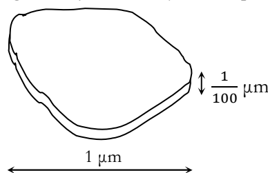
Figure 2.15 : Feuillet d'argile
