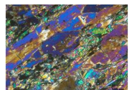
texture nématoblastique
