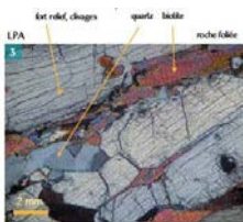
Disthène
