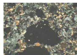
Texture porphyroblastique
