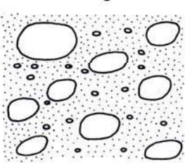
(d) Paraconglomerate
