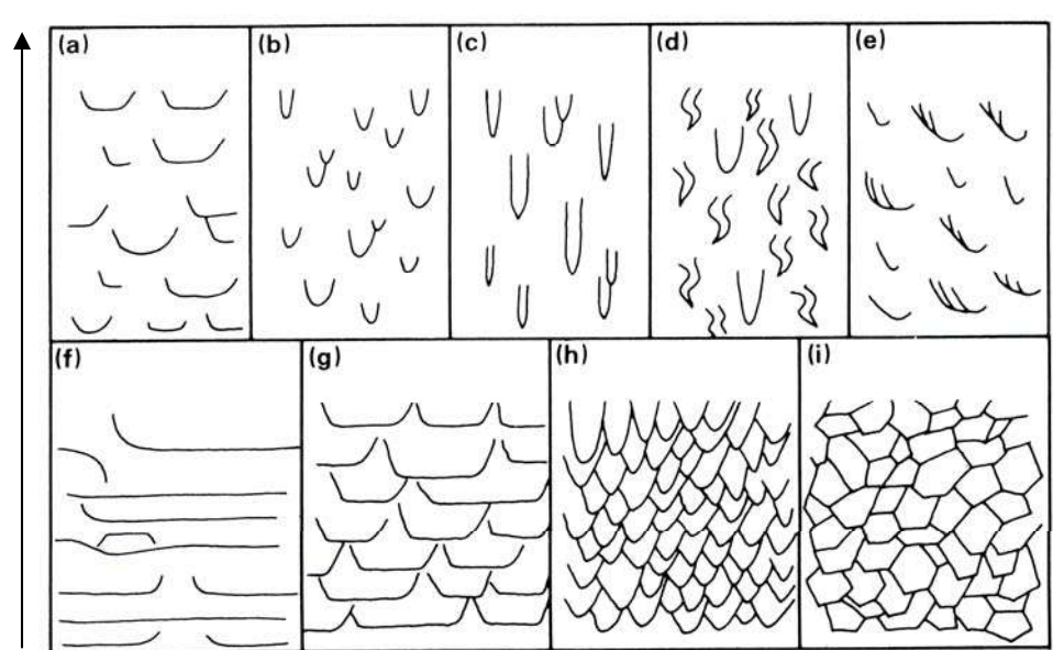
Formes de flutes pour une vue en plan (Allen 1971)
