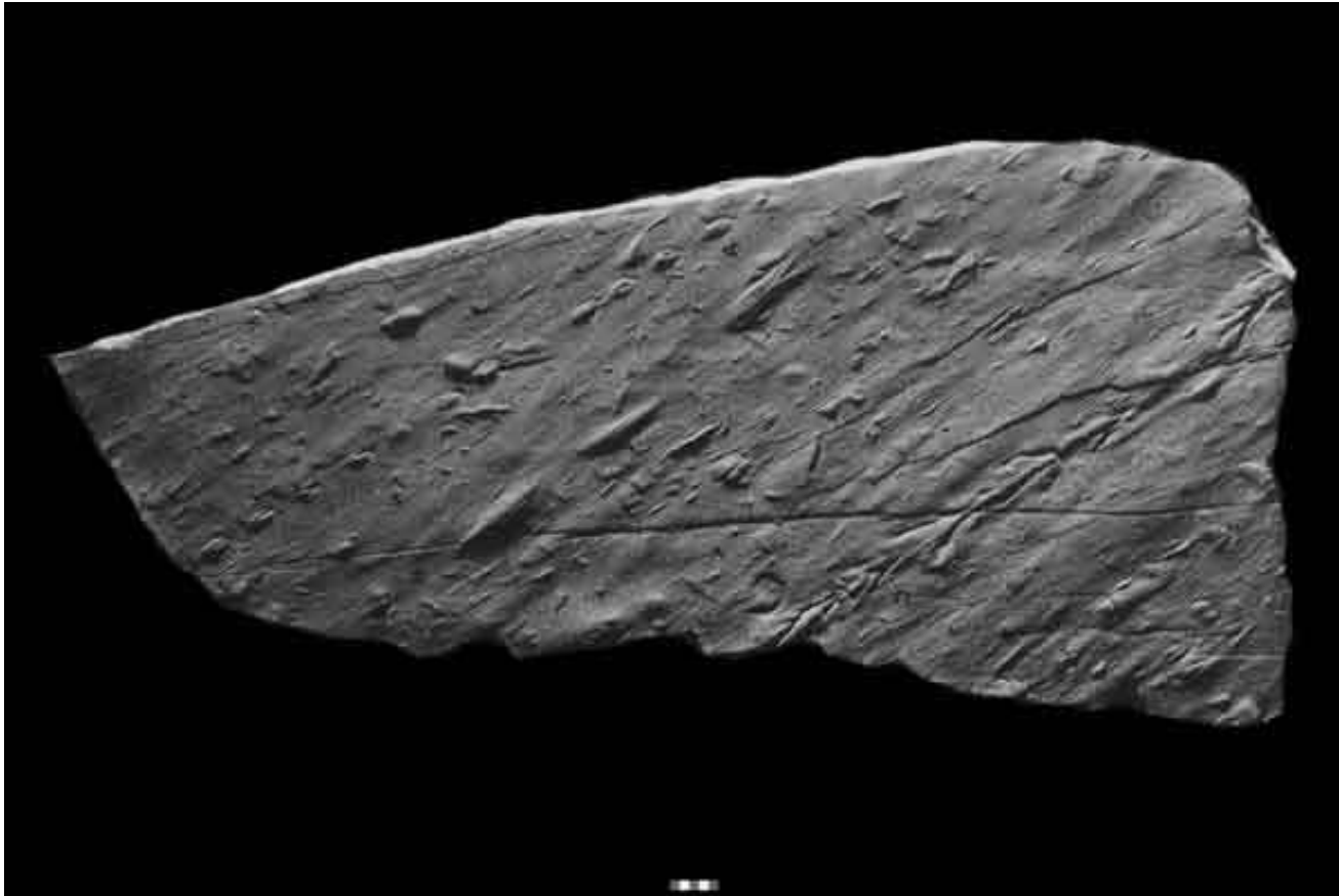
Base d'un banc de grès, assemblage de tool marks: skip, bounce marks, chevron mark. Krosno beds. Oligocene. Kały, Pologne
