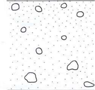
(d) Unstratified unit
