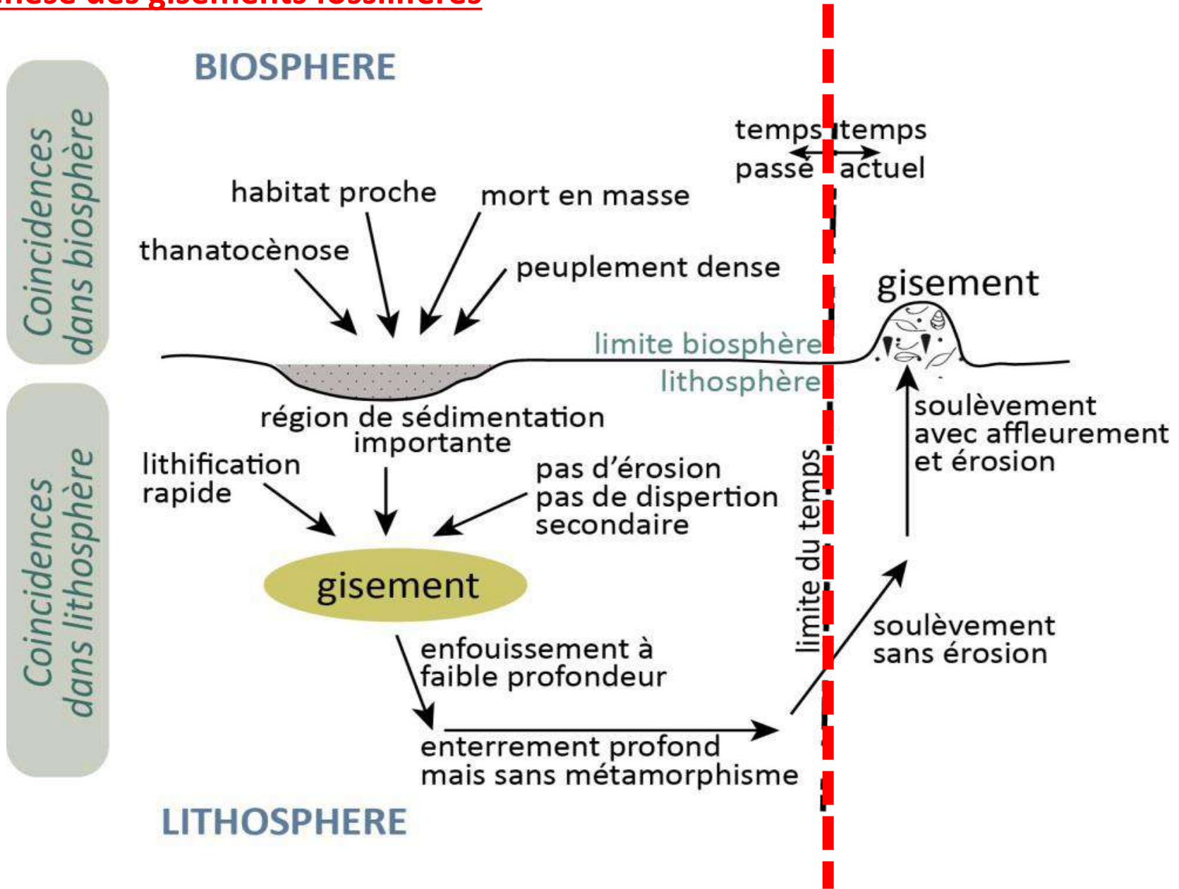
Cycle de formation théorique des gisements fossilifères
