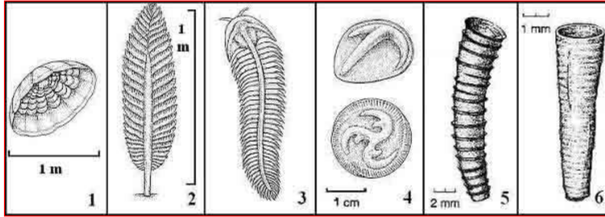
Fossiles de la faune d'Ediacara
