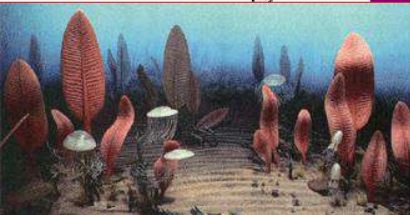
Reconstitution du paléomilieu de la faune d'Ediacara
