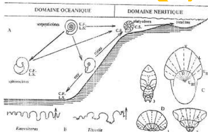
5.27. Signification morphologique nouvelle des cloisons. A. Modèle interprétatif des caractères de la coquille des Ammonoïdes (forme générale, ornementation, espacement, force et complexité des cloisons) et de leur mode de vie. B. Sutures pseudogoniatitiques de Kueniceras ( Engonoceras , Albien) et paradoxocratitiques de Tibotia ( Tissotia , Comiacien-Santonien). C. Vue frontale de la cloison de Macrocephalites à support central (axe des lobes en tireté, des selles en trait plein). D. Différentes formes à support central ; les axes des lobes et des selles reposent : 1, sur des éléments homologues des cloisons du tour précédent ; 2, sur des éléments homologues ou différents ; 3, seulement sur des éléments non homologues (D'après Wright (B), in Moore, 1957 ; Westermann, 1958 (C, D) ; Tintant et al. 1982 ; Ward et Westermann, 1985 (A)). CP = cloisonnement fort (cloisons serrées, très plissées), CS = cloisonnement faible (cloisons espacées et simplifiées). (ENRY, 1990)
