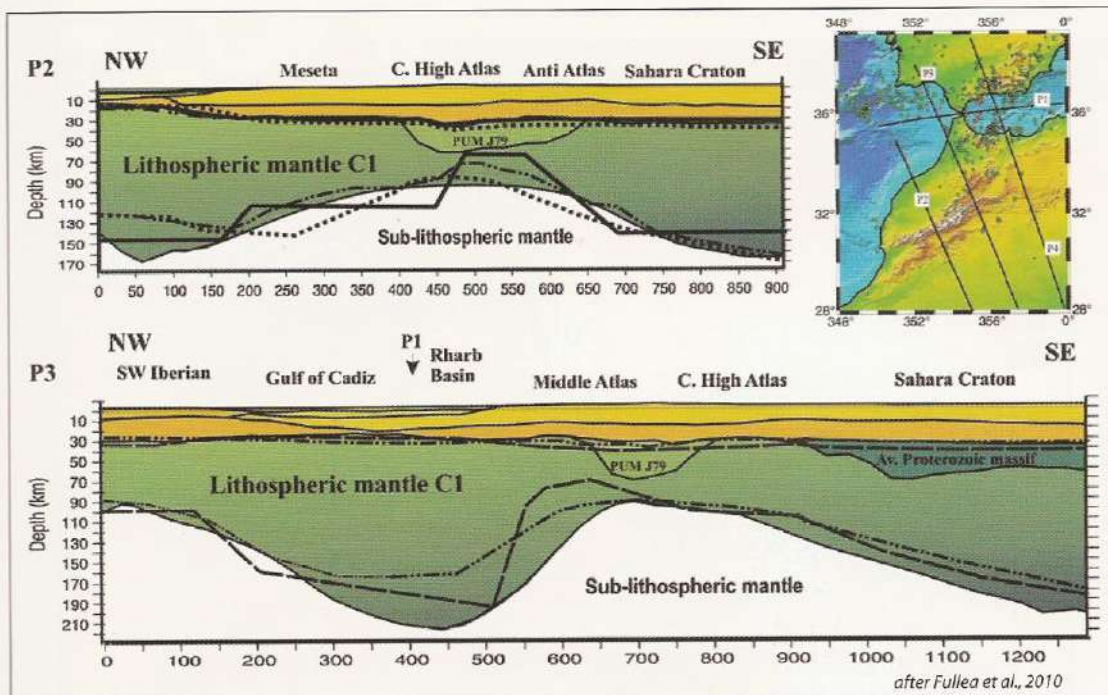
FIG. 4 : Modélisation géophysique de l'anomalie lithosphérique chaude du Maroc, illustrée par deux profils NW-SE (Fullea et al. , 2010). Les traits pointillés et/ou tiretés représentent des solutions antérieurement proposées. Densités adoptées : PUM J79 : Primitive Upper Mantle (référence J79) ; Av. Proterozoic massif : Average etc.
