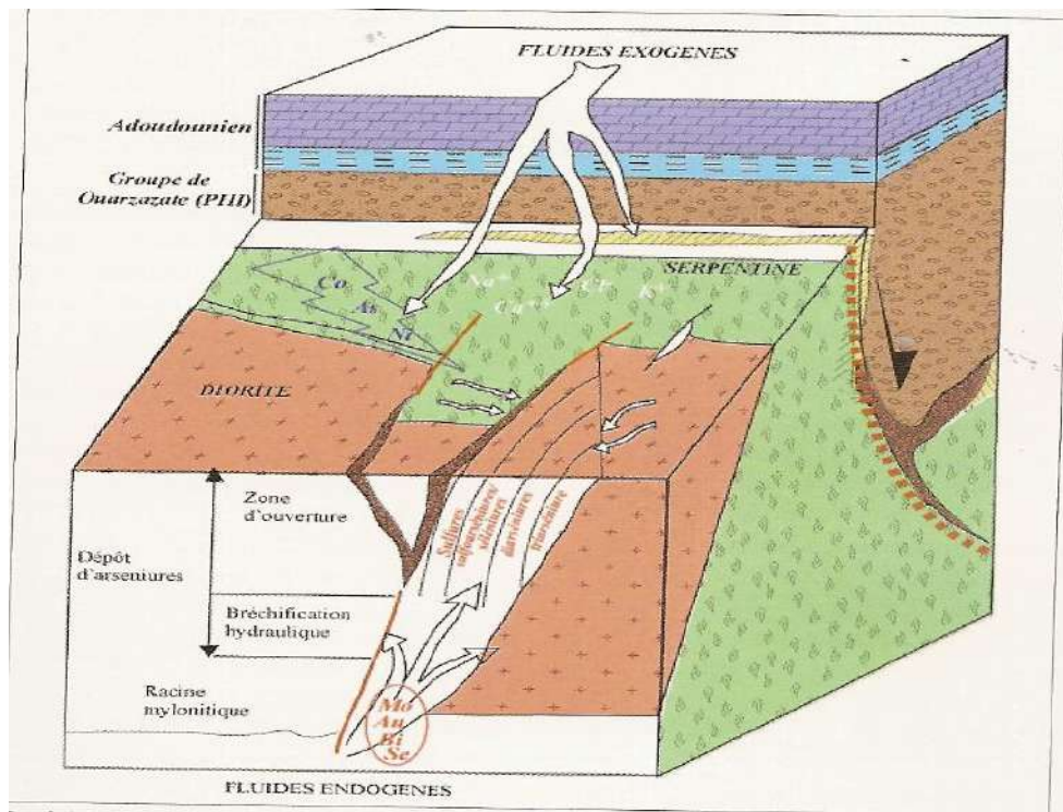
Fig. 2.4.5 : Essai d'interprétations des minéralisations cobaltifères de Bou Azzer (Maacha, 1994, modifié).
