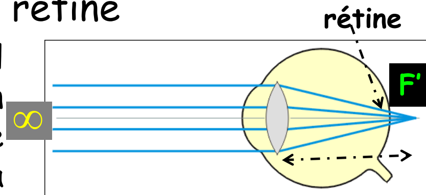
L'œil hypermétrope
