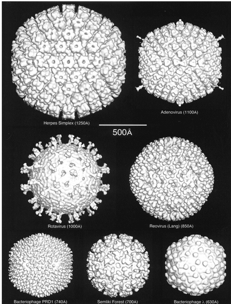
Exemples de virus icosaédriques en Cryo EM (1) 1Angström = 10^{-10} m
