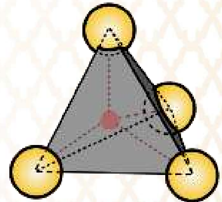
Le tétraèdre de base
