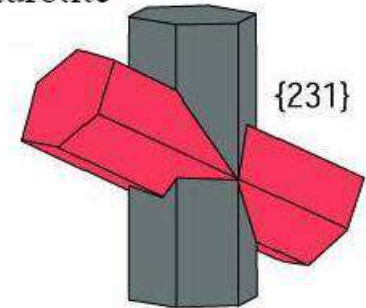
Mâcles de staurotite
