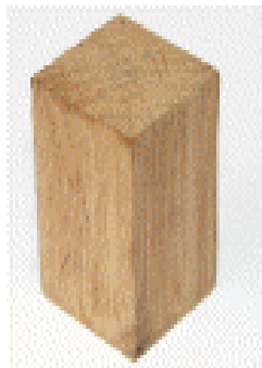
QUADRATIQUE
