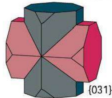
Mâcles de staurotite
