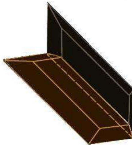
MACLE EN QUEUE D'ARONDE
