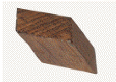
RHOMBOHEDRIQUE
