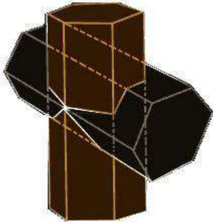
MACLE PAR PENETRATION
