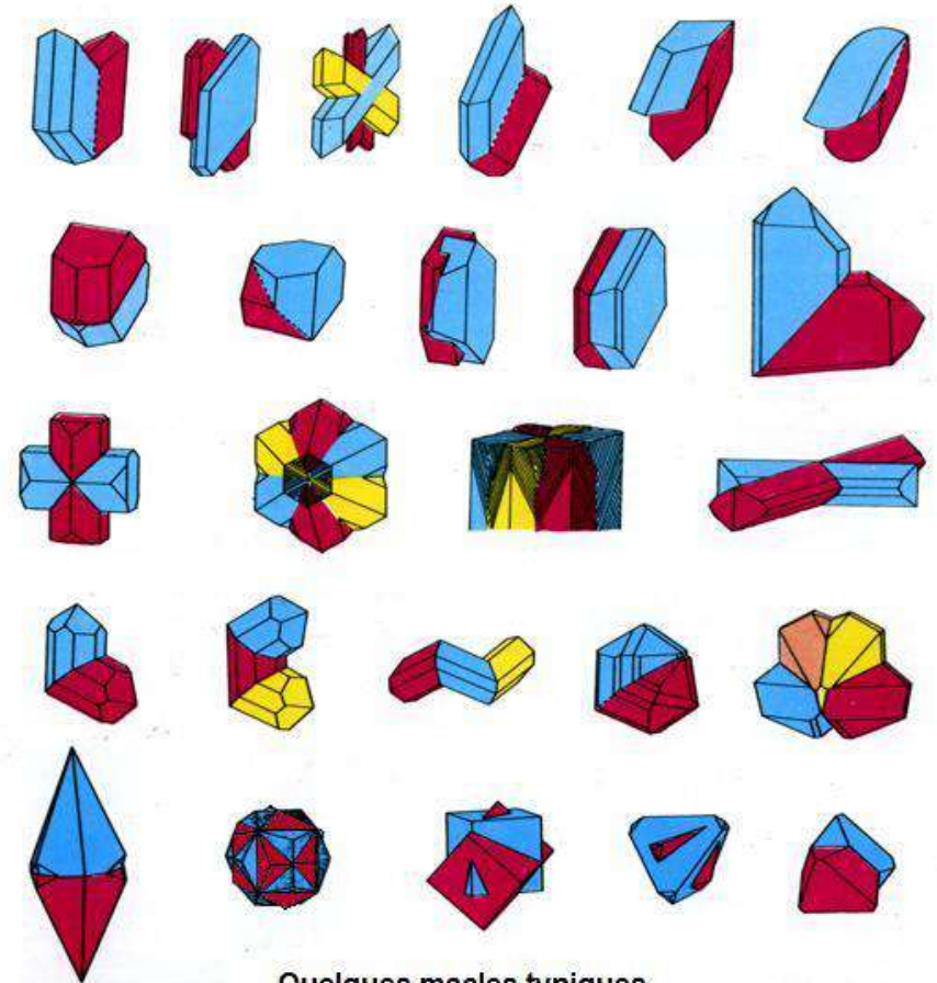
Quelques macles typiques
