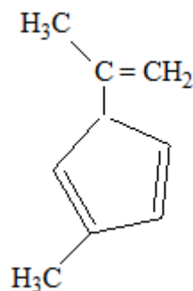
5-isoprényl,3-méthylcyclopenta-1,3-diène
