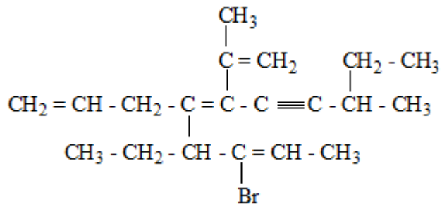
5-allyl,3-bromo,4-éthyl,6-isoprényl,9-méthylundéca-2,5-dièn-7-yne
