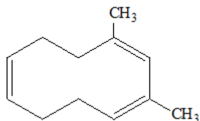
1,3-diméthylcycloclodéca1,3,7-triène
