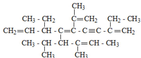
6-(1-éthylallyl)5-isoprényl,7-isopropyldéca-1,5,8-trièn-3-yne
