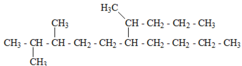
6-(1-méthylbutyl)2,3-diméthyldécane
