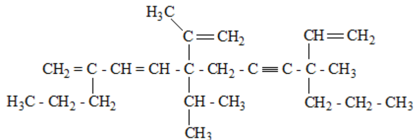
5-isoprényl,5-isopropyl,9-méthyl,2,9-dipropyldéca-1,3,10-trièn-7-yne
