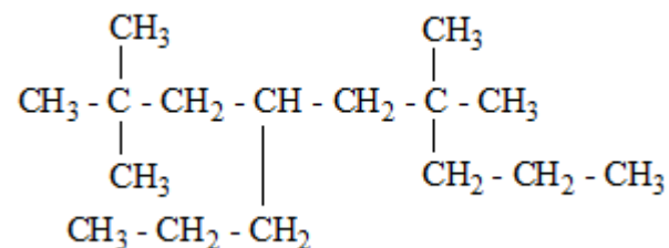
4,4-diméthyl,6-néopentylnonane
