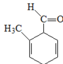
1-méthylcyclohexa-1,4-diène-carbaldéhyde
