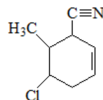
5-chloro,6-méthylcyclohex-2-èncarbonitrile
