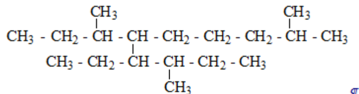
6-éthyl,4,4-diméthylnonane
