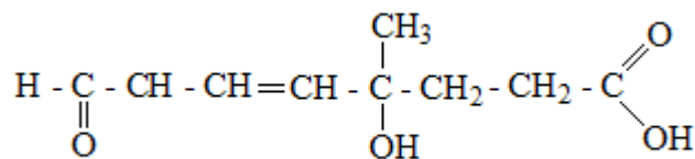
Acide 7-formyl,4-hydroxy,4-méthylhépt-5-énoïque
