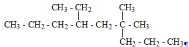
6-éthyl,4,4-diméthylnonane
