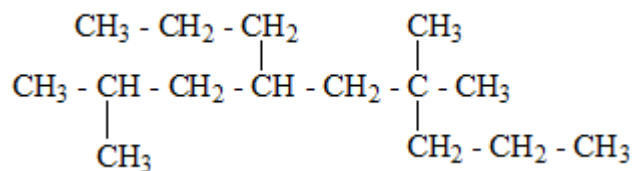
4,4,8-triméthyl,6-propylnonane
