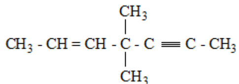
4,4-diméthylhépt-2-èn-5-yne
