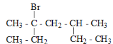
3-bromo,3,5-diméthylhéptane
