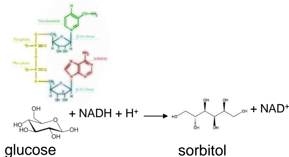
Ex Nicotinamide adénine dinucléotide NAD dans l'aldose réductase
