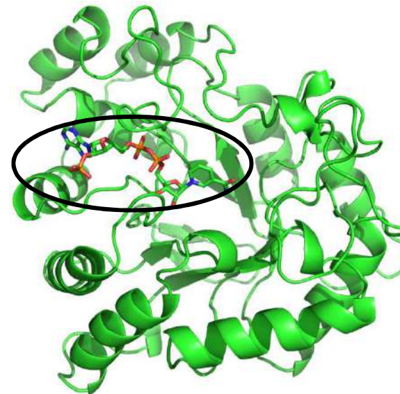
Ex Nicotinamide adénine dinucléotide NAD dans l'aldose réductase
